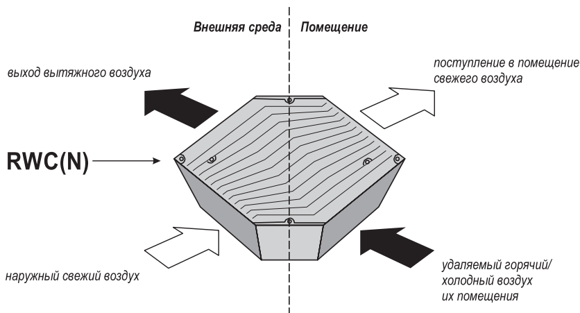
Принцип обмена влажностью
